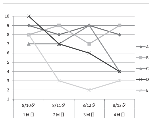
図12. 疲労の変動 (1-10)
