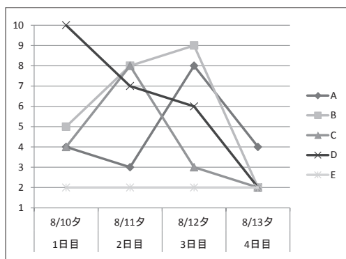
図13. 不安の変動 (1-10)
